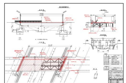
補修設計
